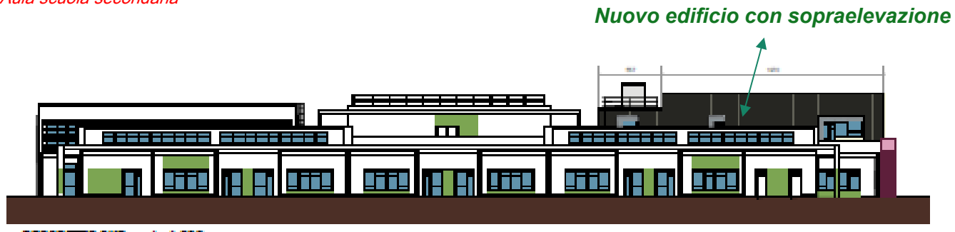
Prospetto sud
